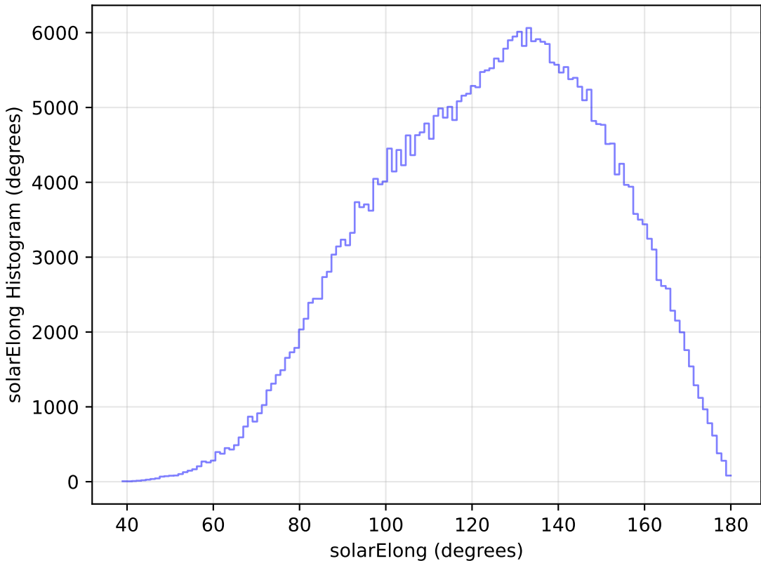
extra_ss_neo3_v3.4_10yrs All sky y band: solarElong Histogram
