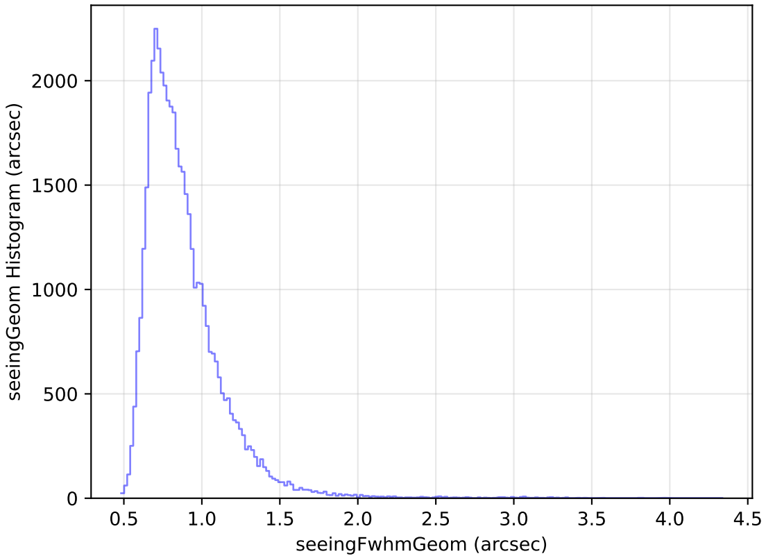
extra_ss_neo3_v3.4_10yrs Yr 1 z band: seeingGeom Histogram
