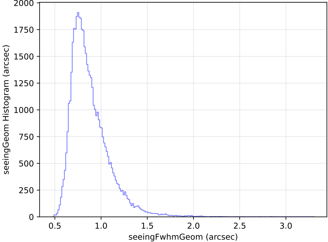
extra_ss_neo3_v3.4_10yrs Yr 1 y band: seeingGeom Histogram
