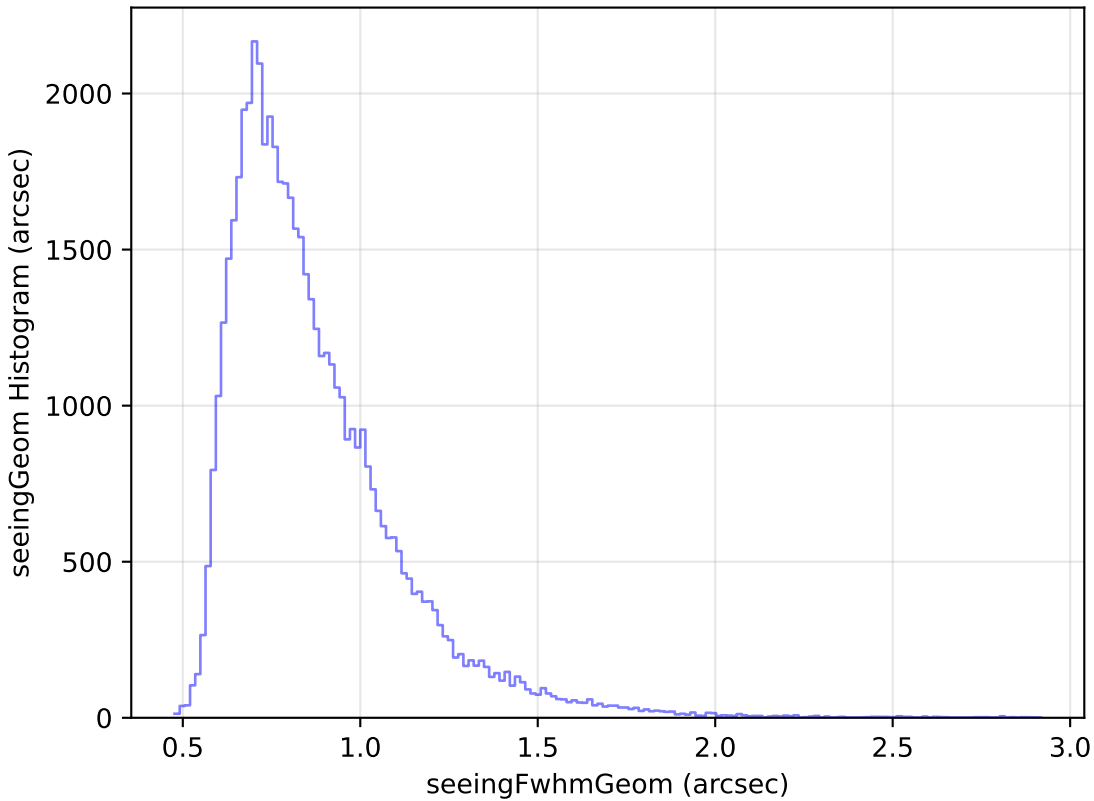
extra_ss_neo3_v3.4_10yrs Yr 1 i band: seeingGeom Histogram
