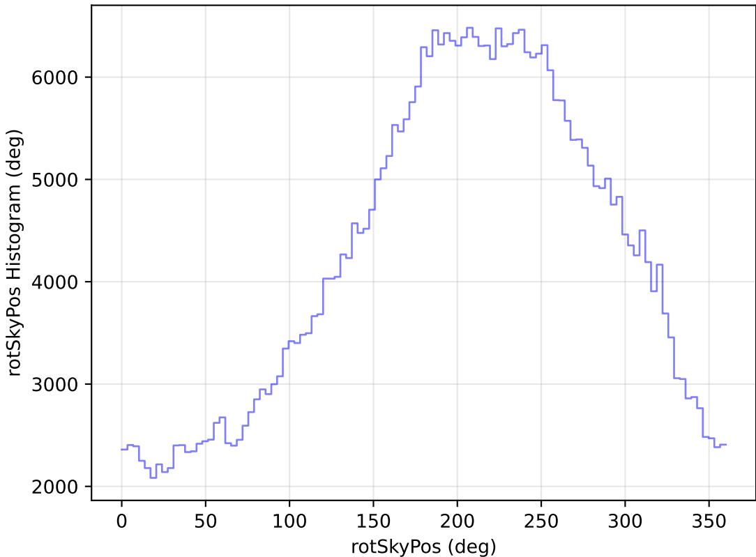
extra_ss_neo3_v3.4_10yrs WFD z band: rotSkyPos Histogram
