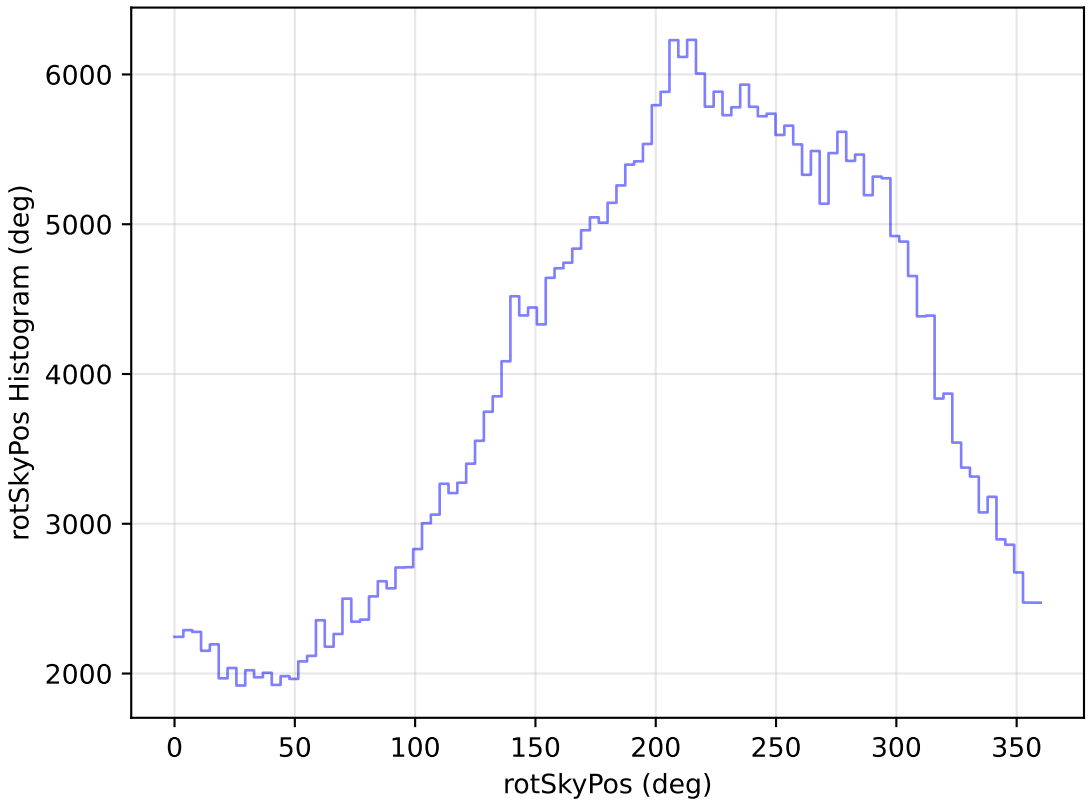
extra_ss_neo3_v3.4_10yrs WFD y band: rotSkyPos Histogram
