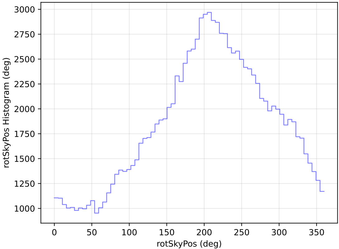
extra_ss_neo3_v3.4_10yrs WFD u band: rotSkyPos Histogram
