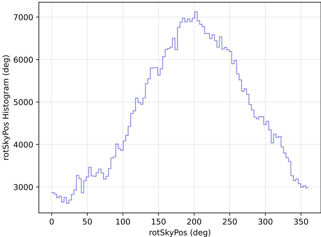
extra_ss_neo3_v3.4_10yrs WFD r band: rotSkyPos Histogram
