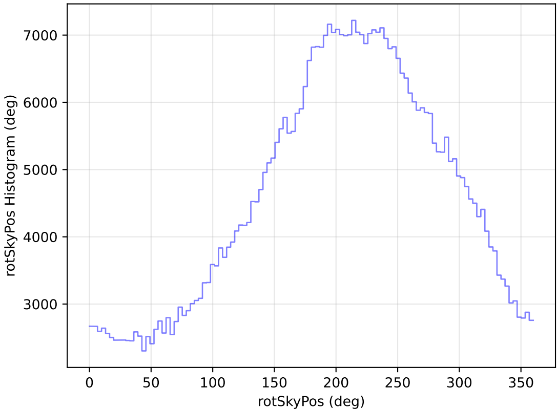
extra_ss_neo3_v3.4_10yrs WFD i band: rotSkyPos Histogram
