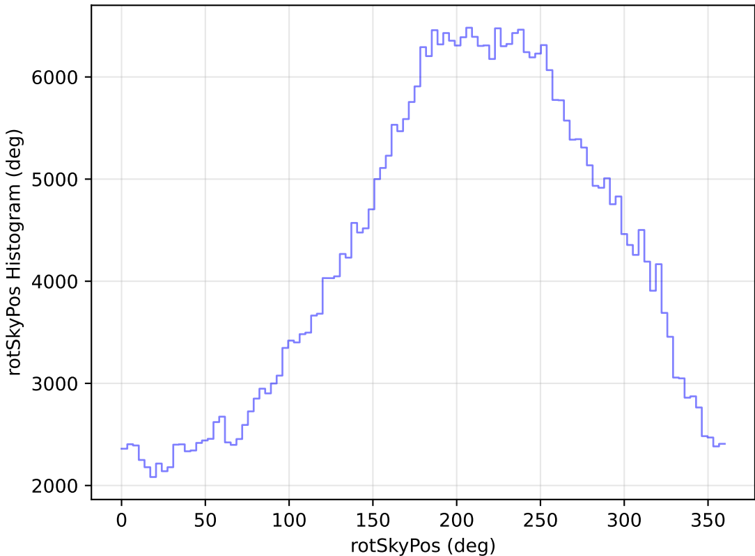
extra_ss_neo3_v3.4_10yrs All sky z band: rotSkyPos Histogram
