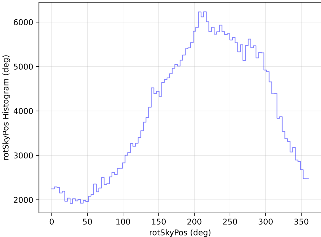
extra_ss_neo3_v3.4_10yrs All sky y band: rotSkyPos Histogram
