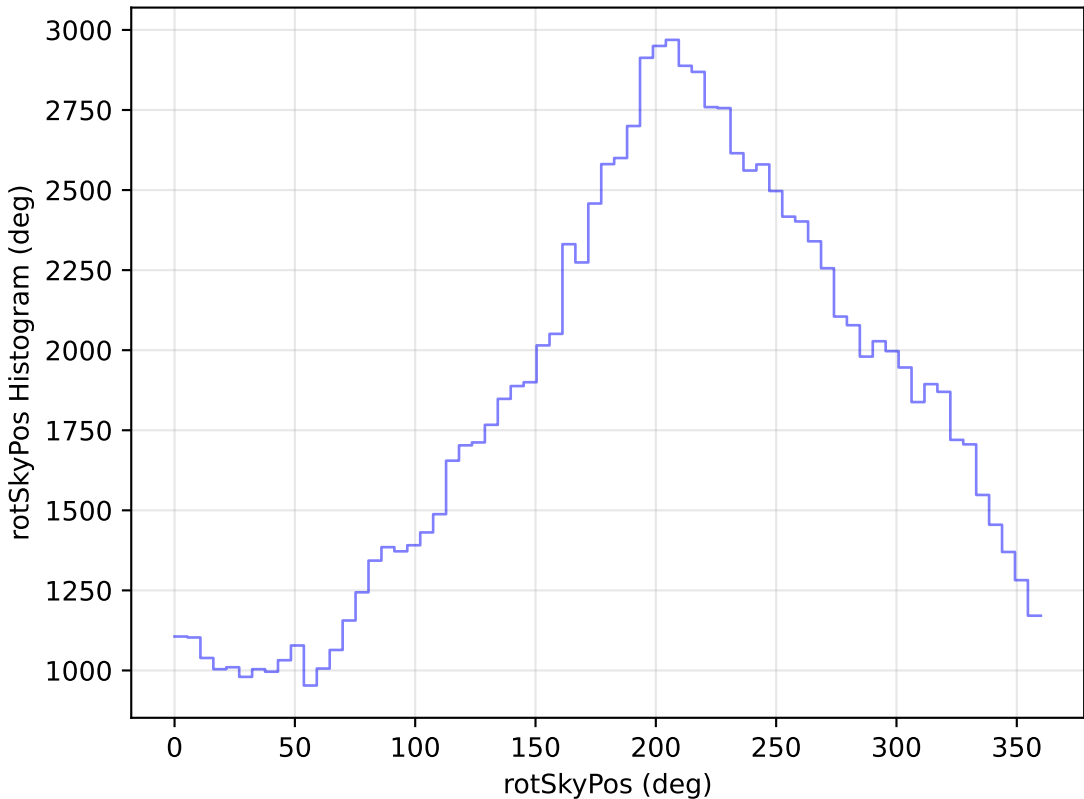
extra_ss_neo3_v3.4_10yrs All sky u band: rotSkyPos Histogram
