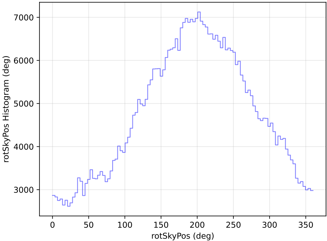
extra_ss_neo3_v3.4_10yrs All sky r band: rotSkyPos Histogram
