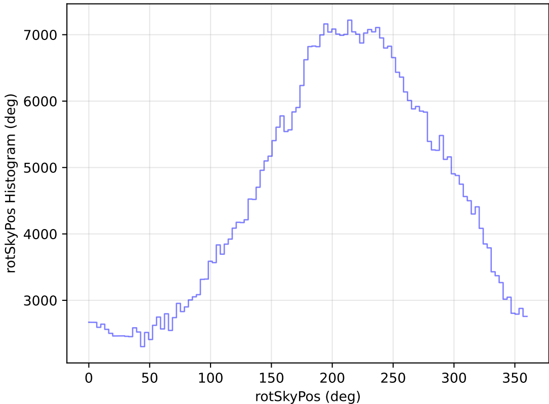
extra_ss_neo3_v3.4_10yrs All sky i band: rotSkyPos Histogram
