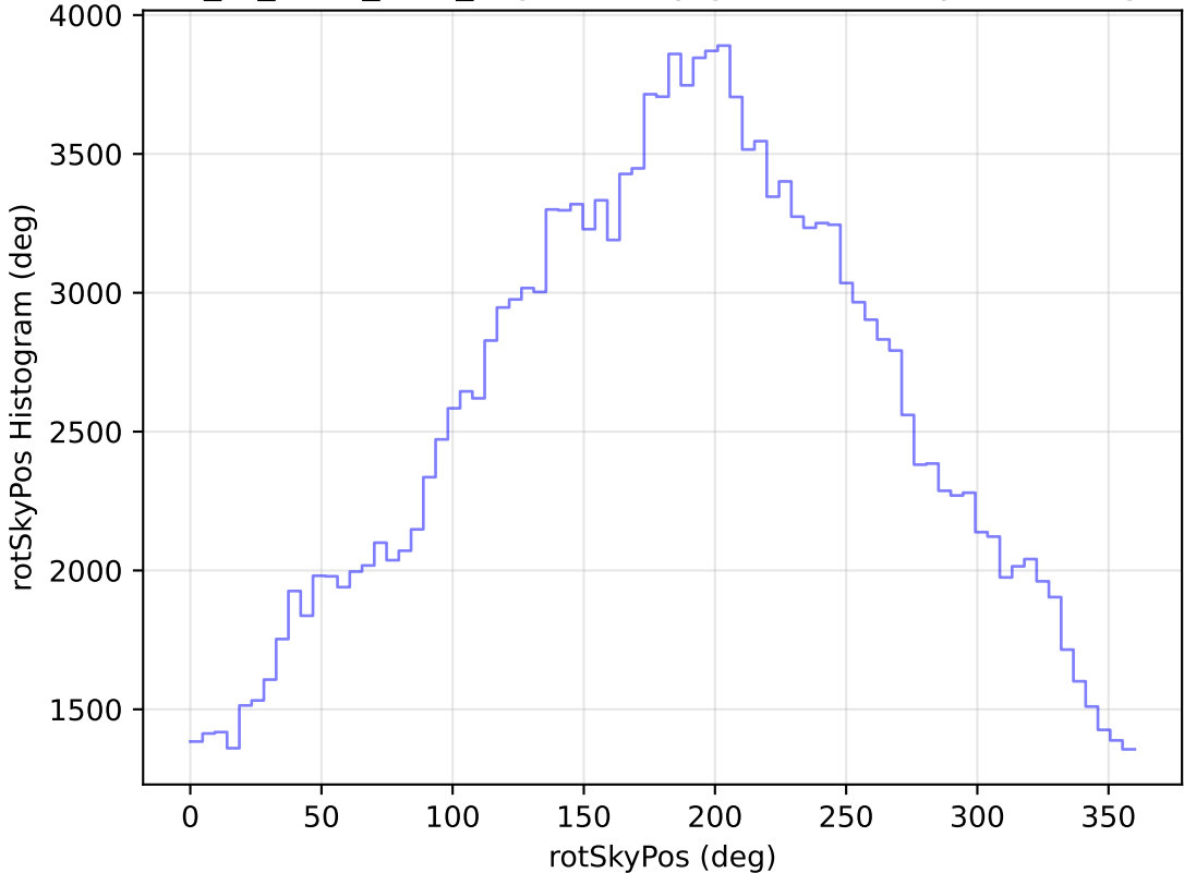
extra_ss_neo3_v3.4_10yrs All sky g band: rotSkyPos Histogram
