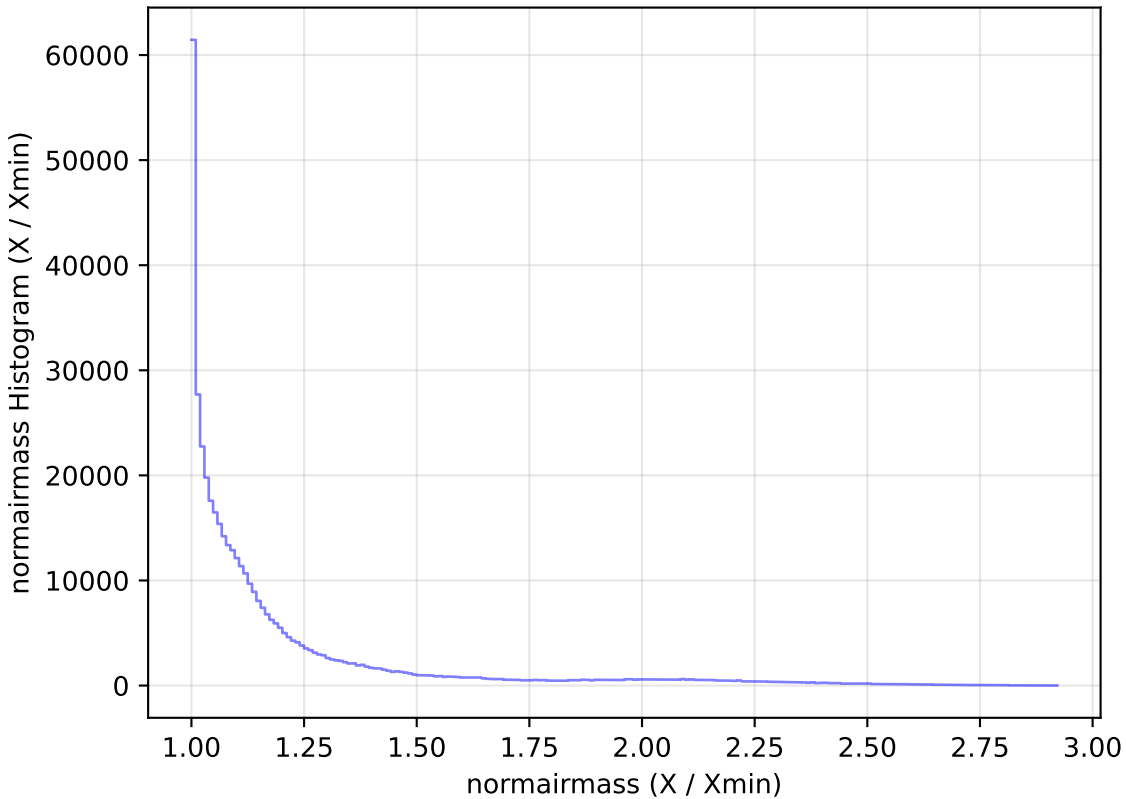
extra_ss_neo3_v3.4_10yrs All sky z band: normairmass Histogram
