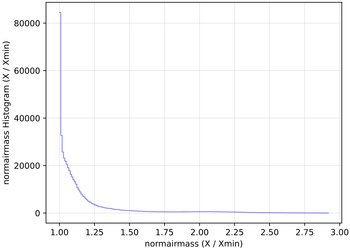
extra_ss_neo3_v3.4_10yrs All sky i band: normairmass Histogram
