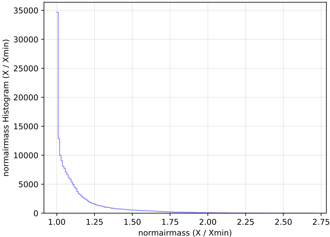
extra_ss_neo3_v3.4_10yrs All sky g band: normairmass Histogram
