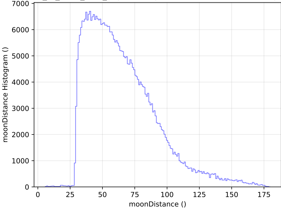
extra_ss_neo3_v3.4_10yrs WFD y band: moonDistance Histogram
