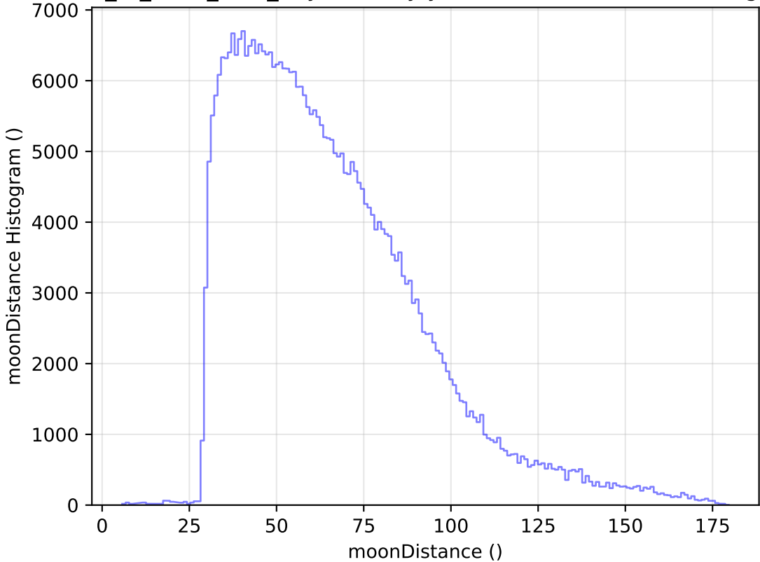
extra_ss_neo3_v3.4_10yrs All sky y band: moonDistance Histogram
