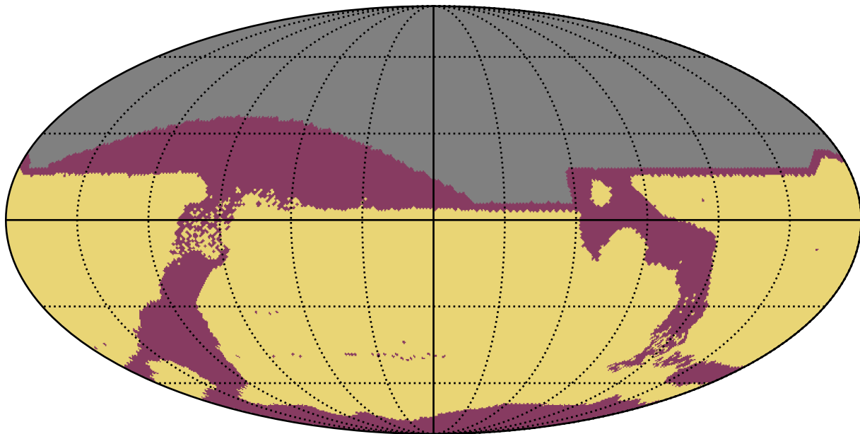
extra_ss_neo3_v3.4_10yrs All sky: RapidRevisits
