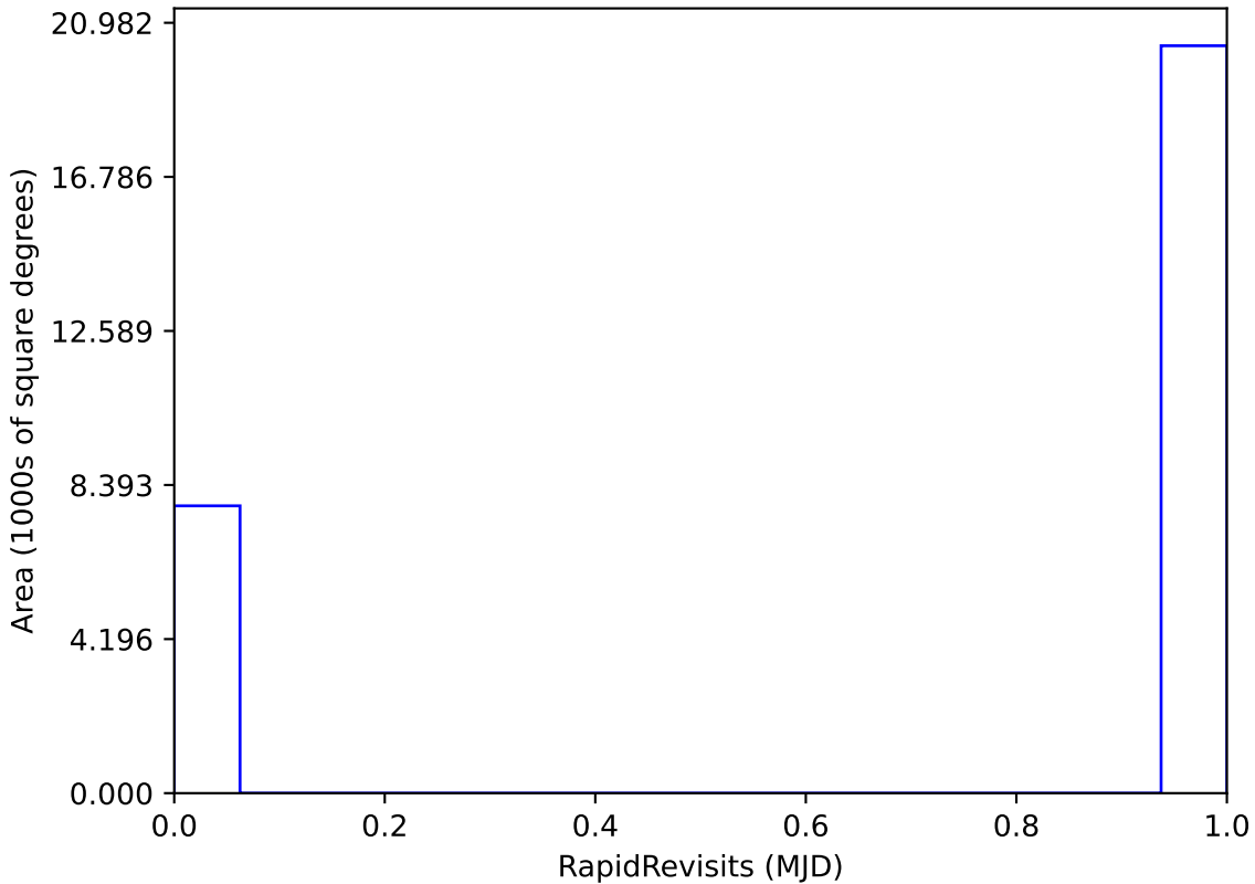
extra_ss_neo3_v3.4_10yrs All sky: RapidRevisits
