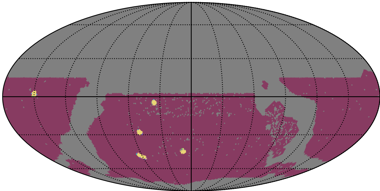
extra_ss_neo3_v3.4_10yrs WFD: NumberOfQuickRevisits
