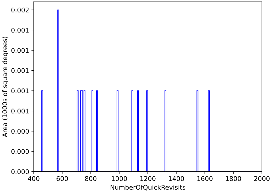
extra_ss_neo3_v3.4_10yrs WFD: NumberOfQuickRevisits
