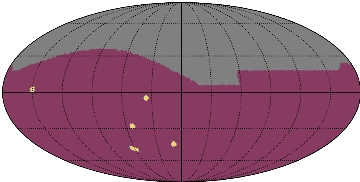
extra_ss_neo3_v3.4_10yrs All sky: NumberOfQuickRevisits
