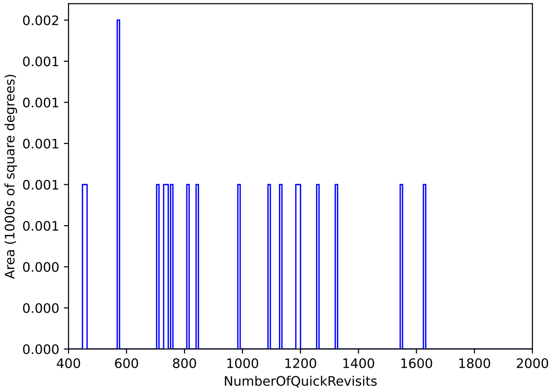
extra_ss_neo3_v3.4_10yrs All sky: NumberOfQuickRevisits
