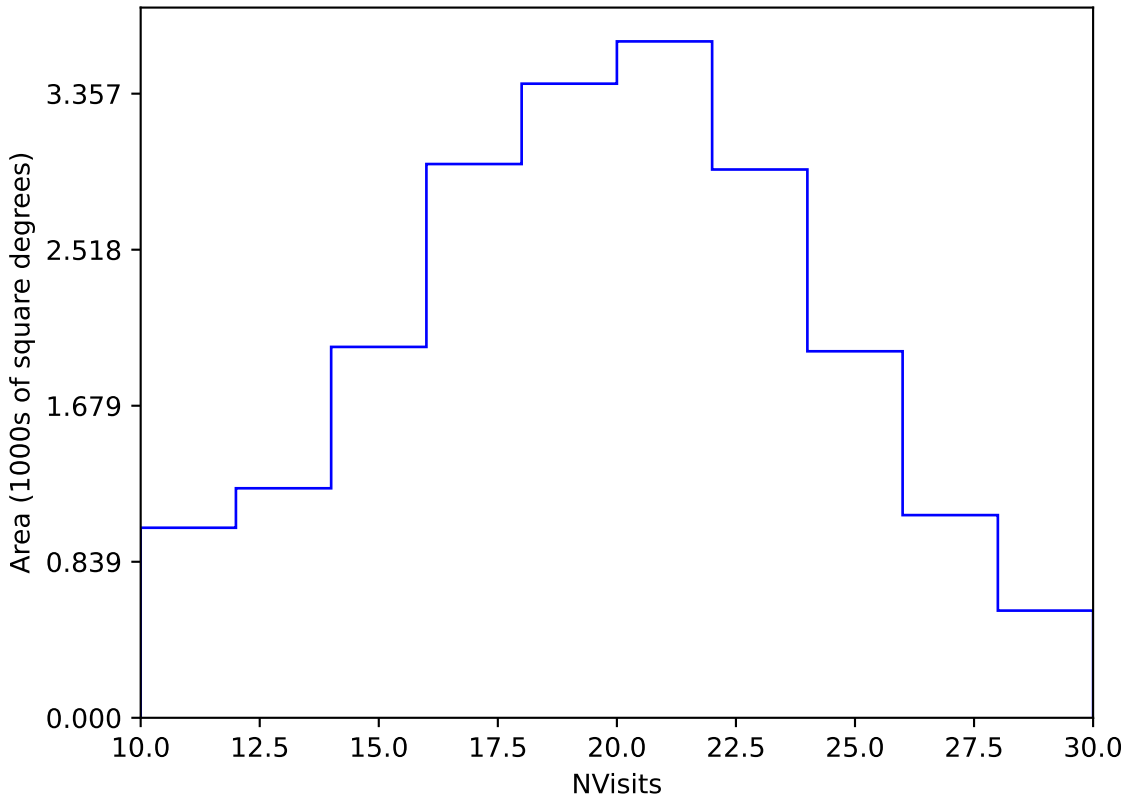
extra_ss_neo3_v3.4_10yrs Yr 1 y band: NVisits
