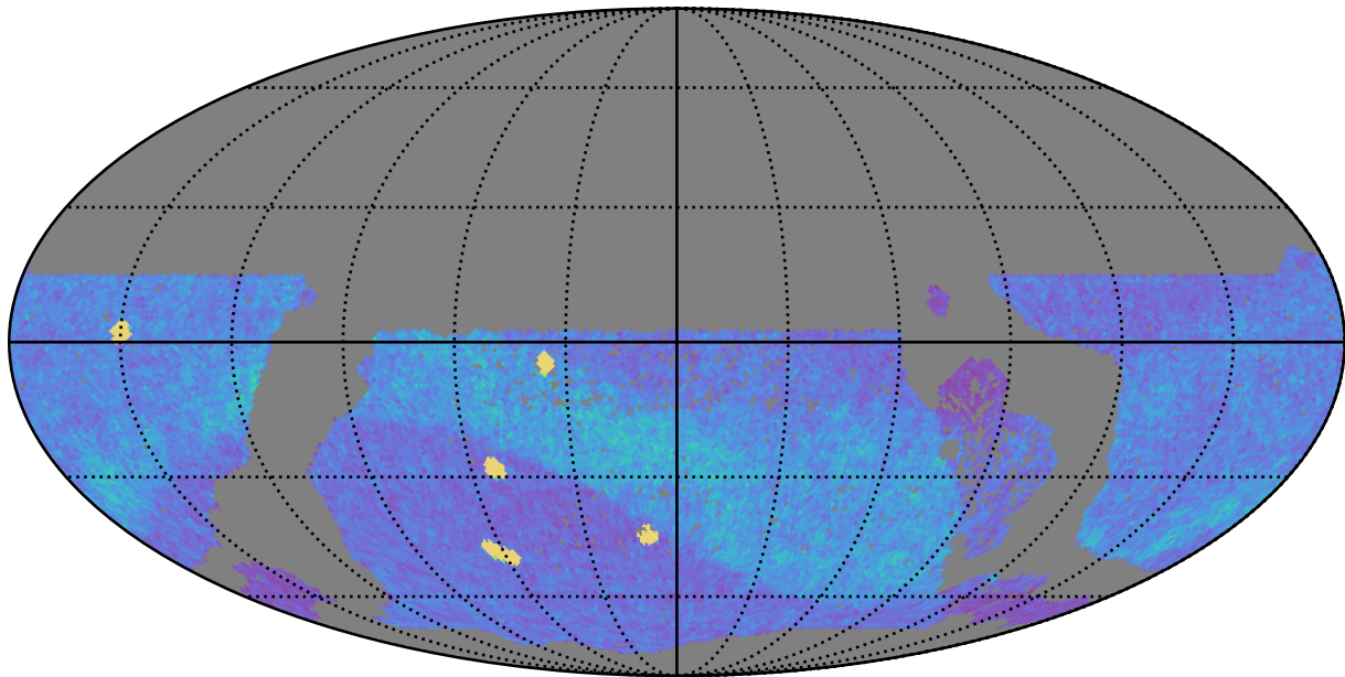
extra_ss_neo3_v3.4_10yrs WFD z band: NVisits
