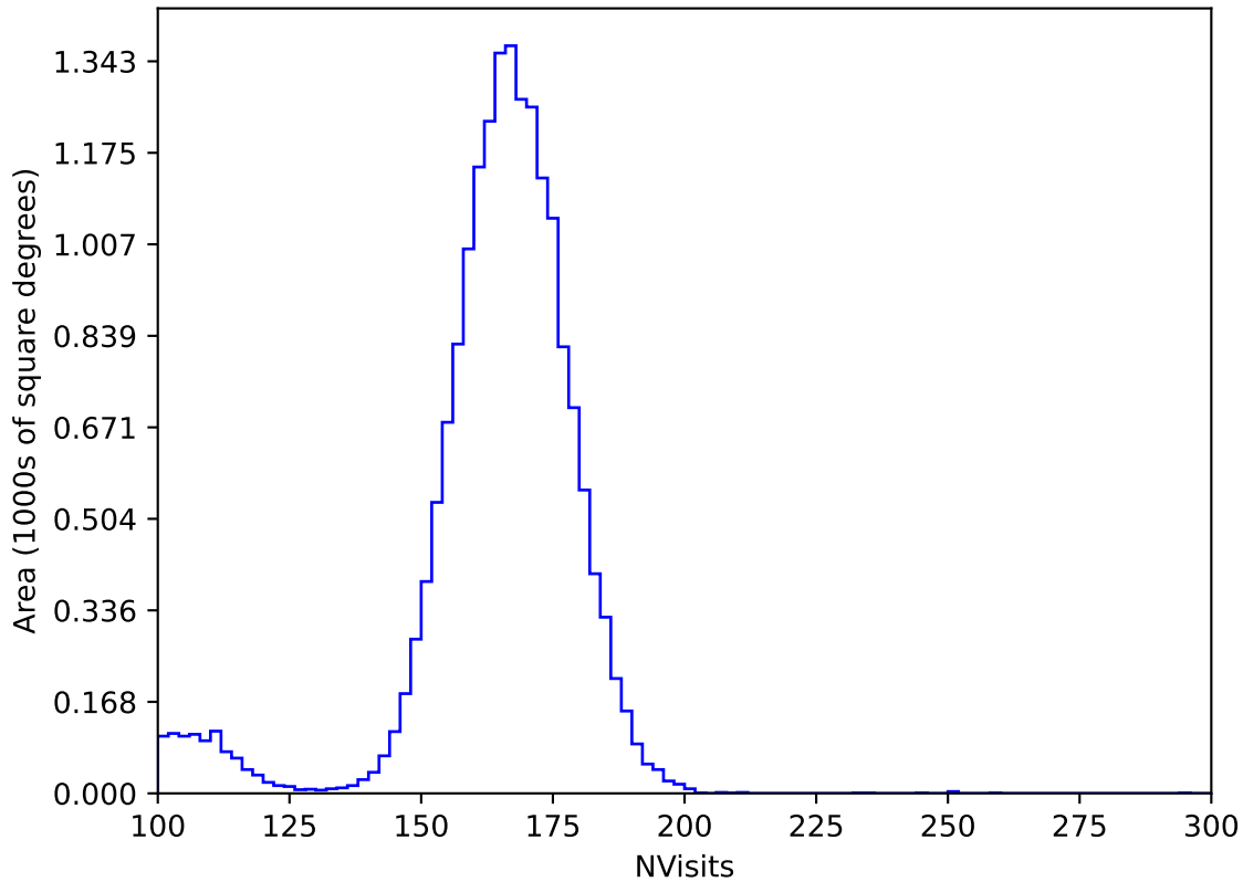
extra_ss_neo3_v3.4_10yrs WFD y band: NVisits
