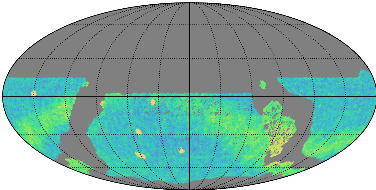
extra_ss_neo3_v3.4_10yrs WFD r band: NVisits
