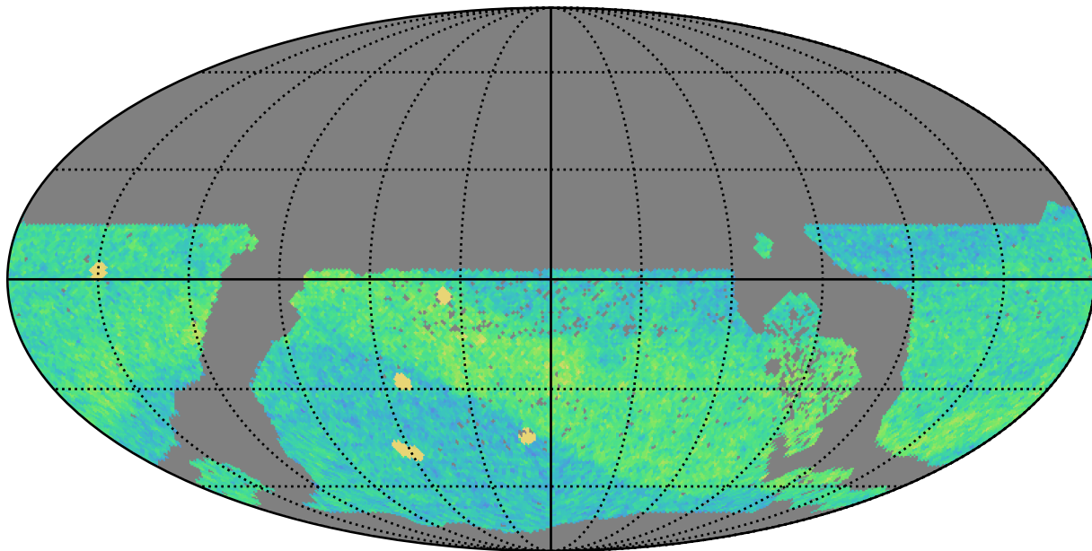
extra_ss_neo3_v3.4_10yrs WFD i band: NVisits
