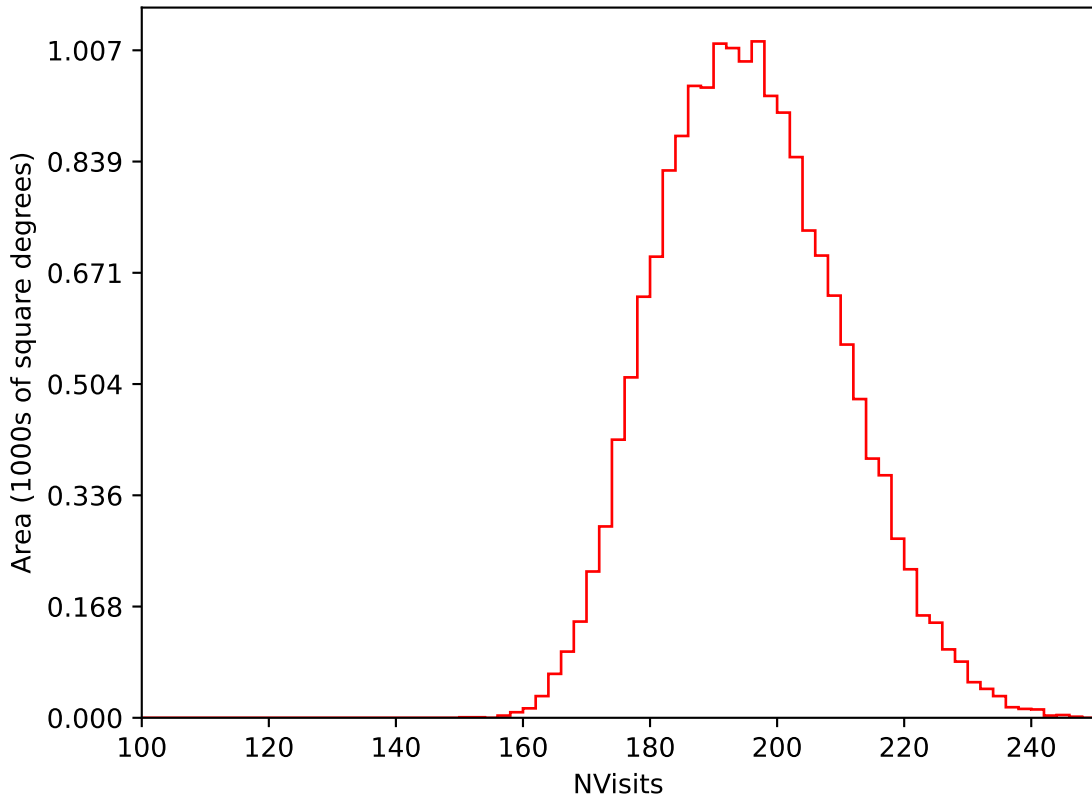
extra_ss_neo3_v3.4_10yrs WFD i band: NVisits
