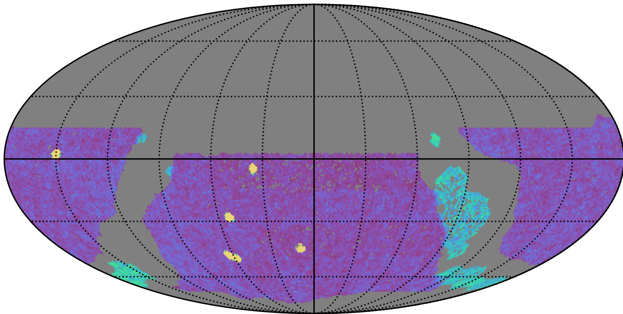
extra_ss_neo3_v3.4_10yrs WFD g band: NVisits
