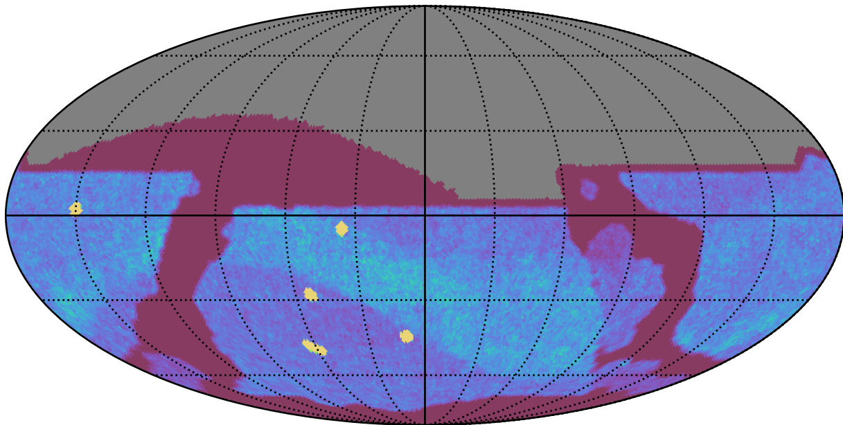
extra_ss_neo3_v3.4_10yrs All sky z band: NVisits
