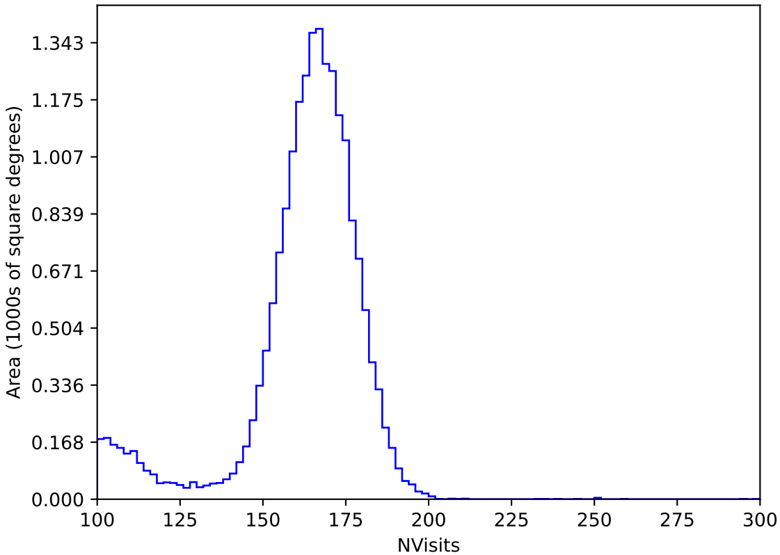
extra_ss_neo3_v3.4_10yrs All sky y band: NVisits
