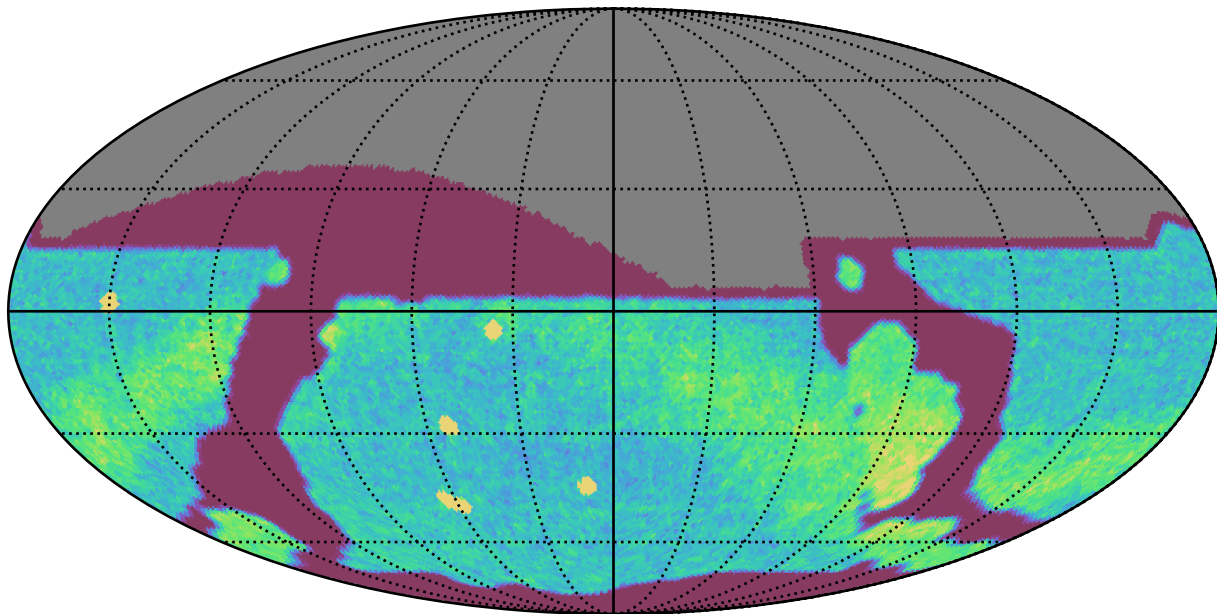
extra_ss_neo3_v3.4_10yrs All sky r band: NVisits
