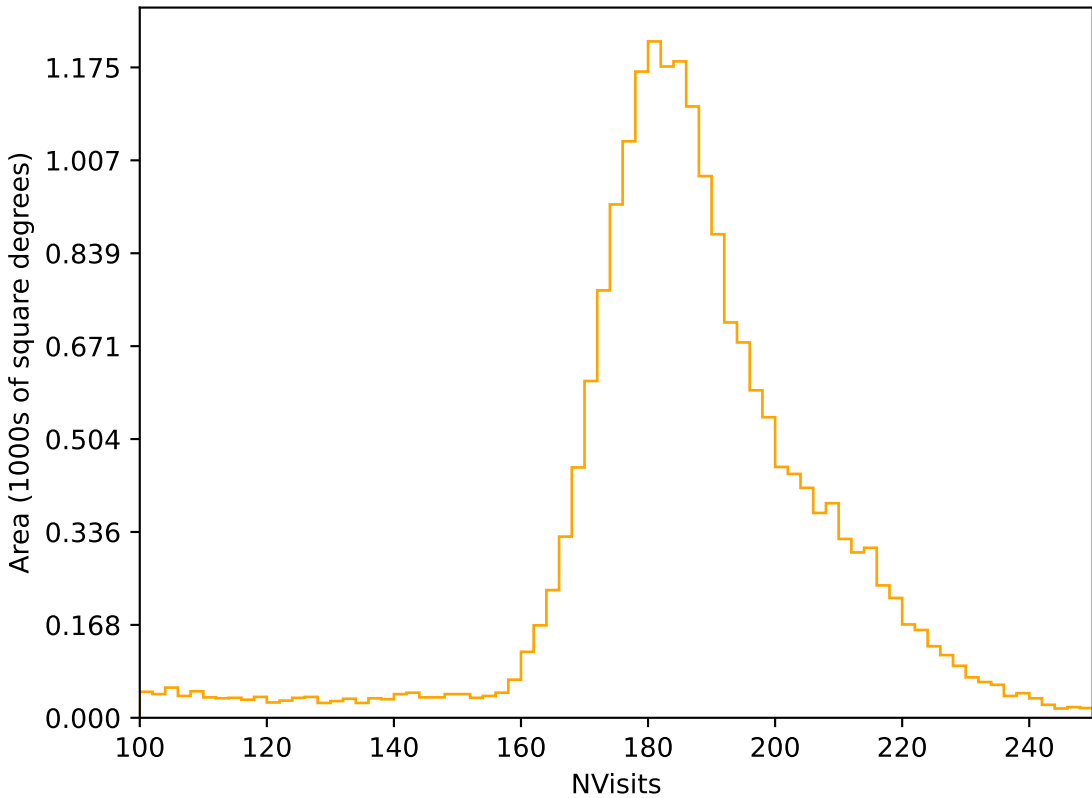
extra_ss_neo3_v3.4_10yrs All sky r band: NVisits
