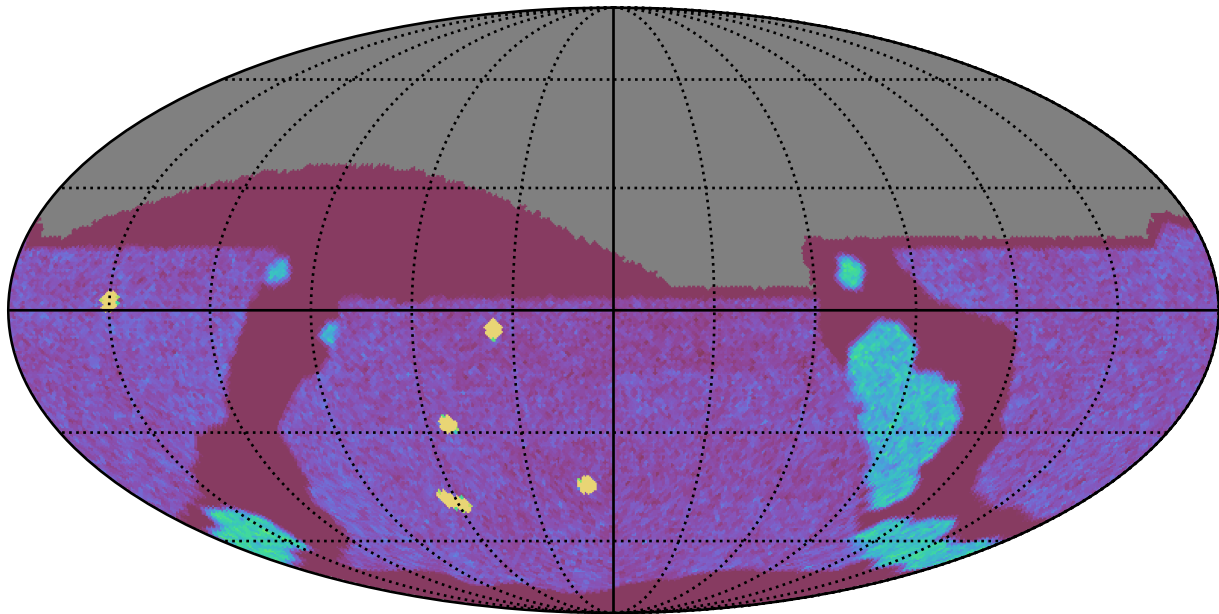
extra_ss_neo3_v3.4_10yrs All sky g band: NVisits
