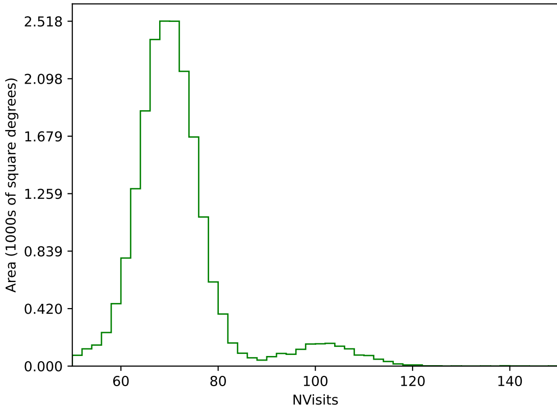
extra_ss_neo3_v3.4_10yrs All sky g band: NVisits
