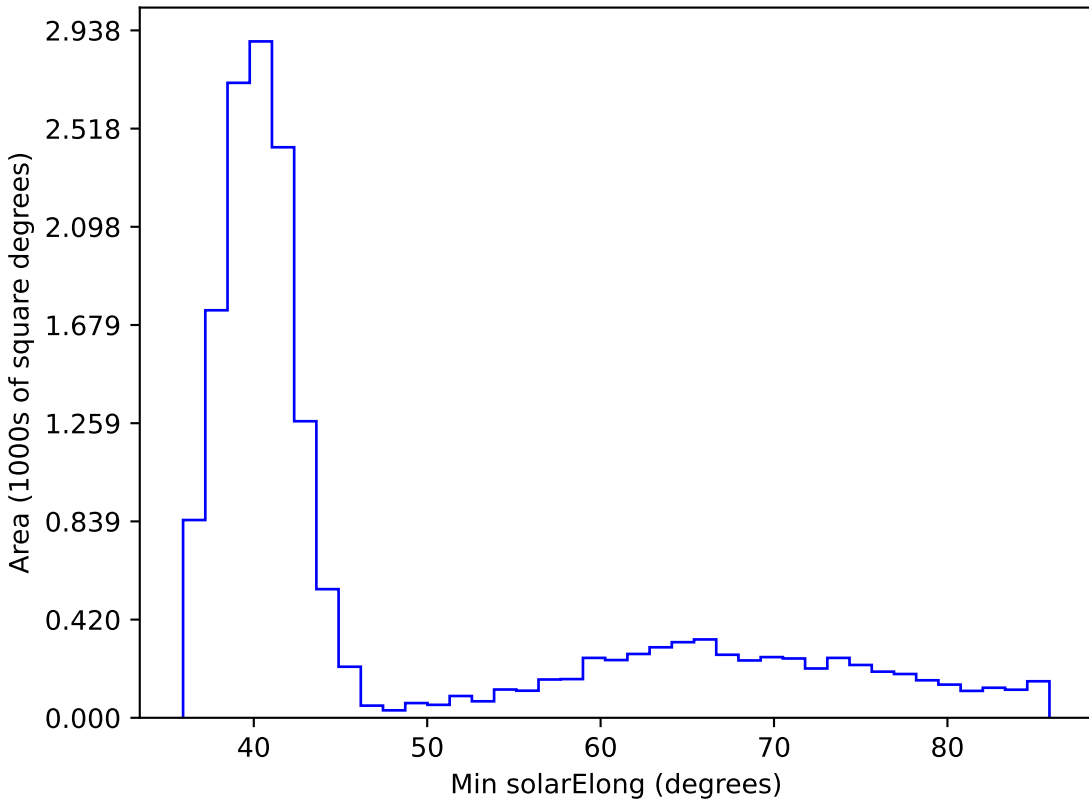
extra_ss_neo3_v3.4_10yrs WFD z band: Min solarElong
