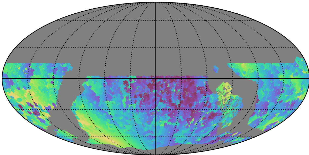
extra_ss_neo3_v3.4_10yrs WFD y band: Min solarElong
