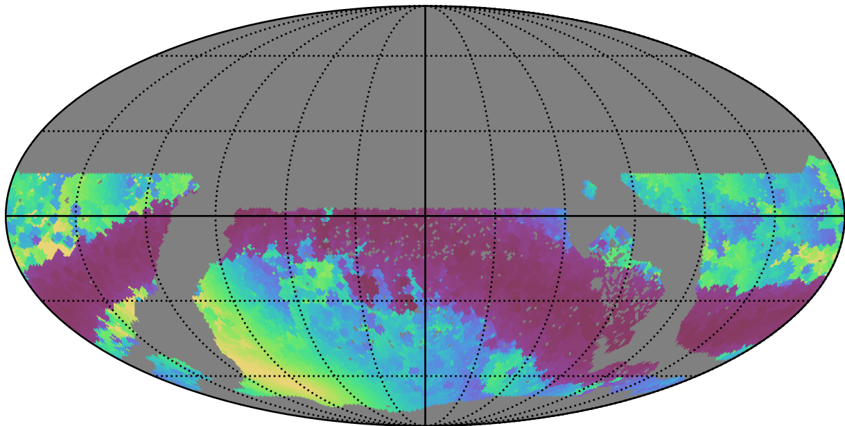
extra_ss_neo3_v3.4_10yrs WFD r band: Min solarElong
