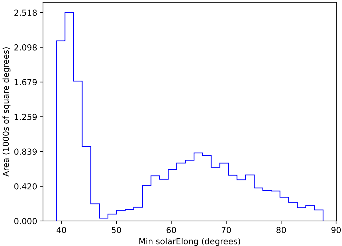
extra_ss_neo3_v3.4_10yrs WFD r band: Min solarElong
