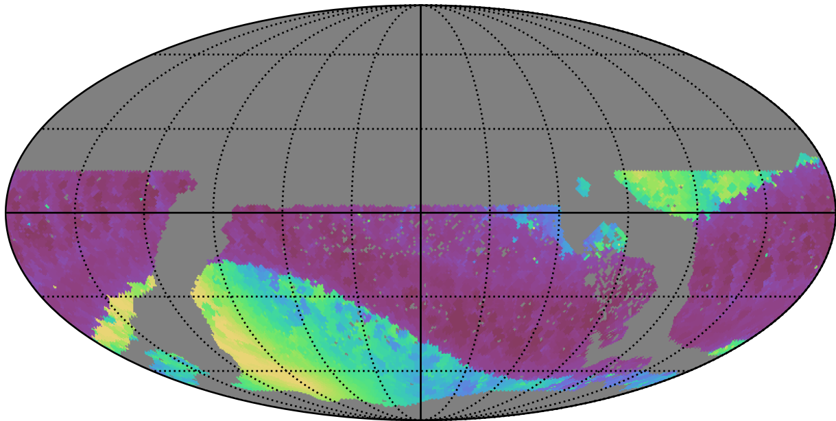
extra_ss_neo3_v3.4_10yrs WFD i band: Min solarElong
