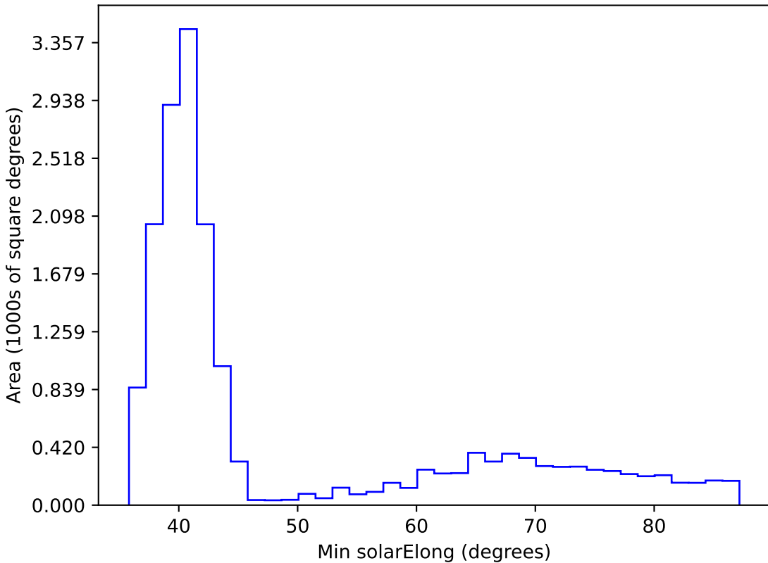
extra_ss_neo3_v3.4_10yrs WFD i band: Min solarElong
