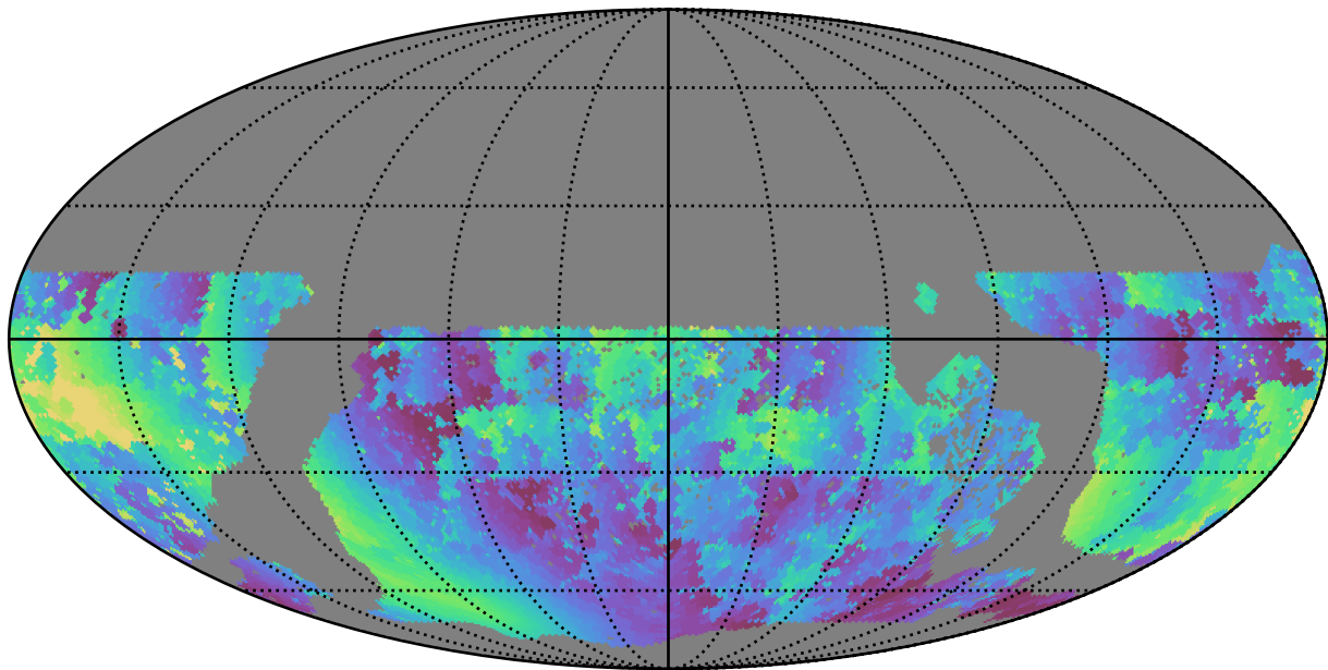
extra_ss_neo3_v3.4_10yrs WFD g band: Min solarElong
