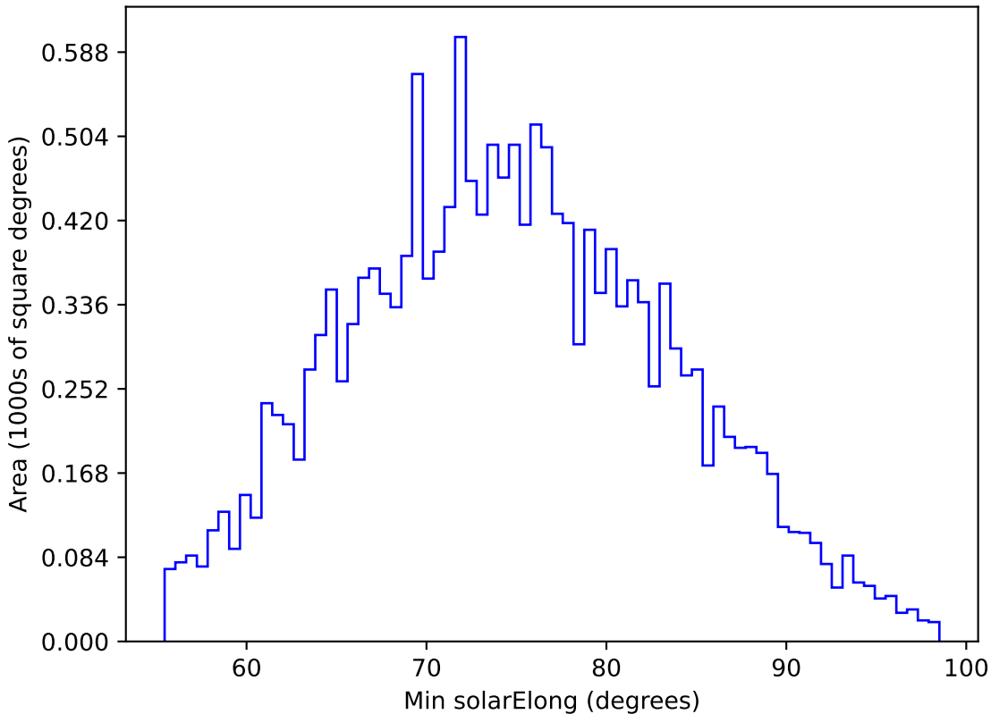
extra_ss_neo3_v3.4_10yrs WFD g band: Min solarElong
