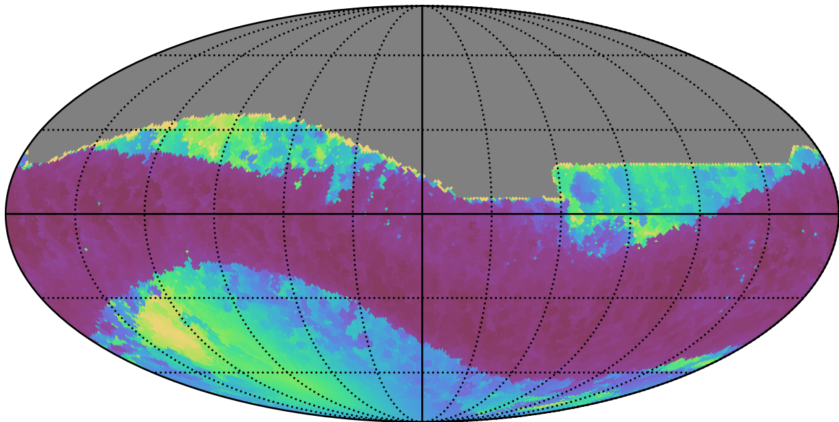
extra_ss_neo3_v3.4_10yrs All sky z band: Min solarElong
