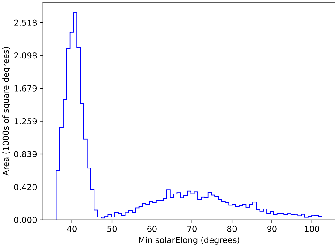
extra_ss_neo3_v3.4_10yrs All sky z band: Min solarElong
