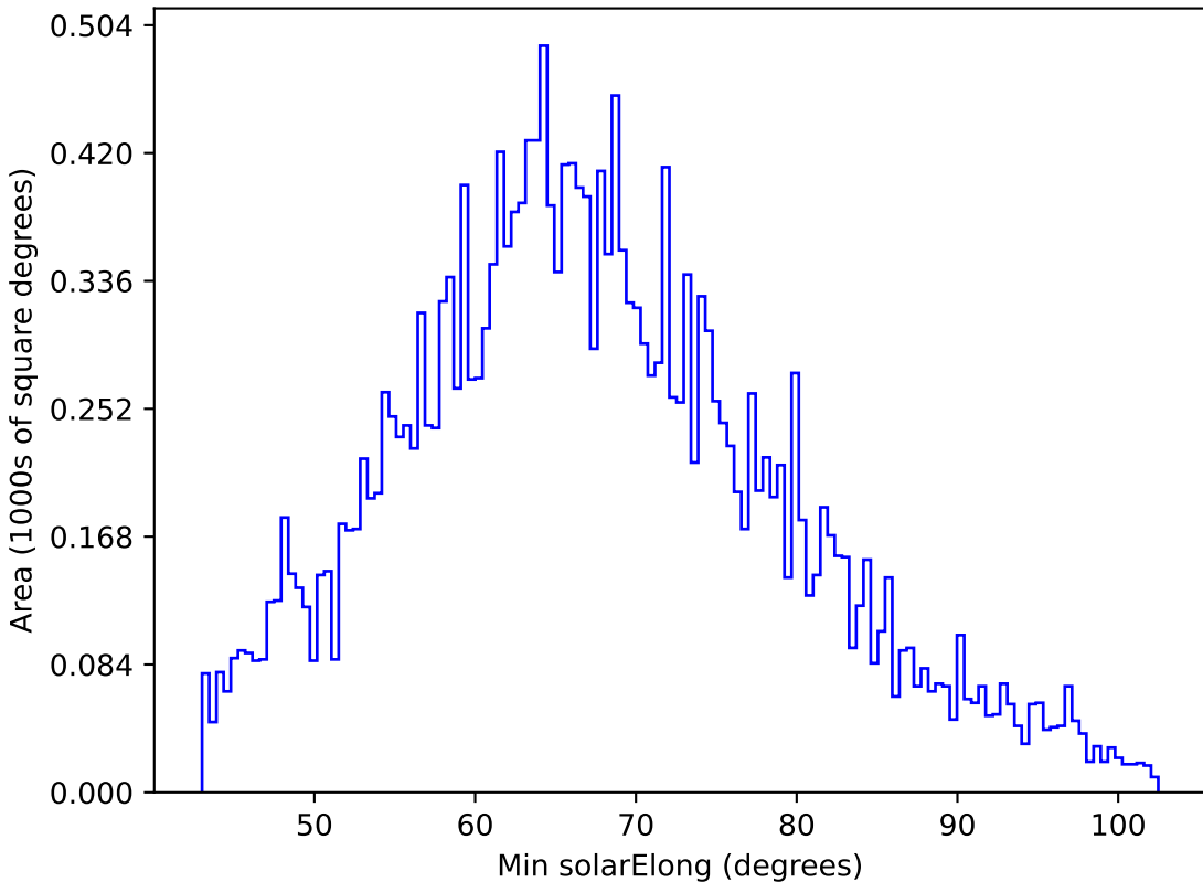
extra_ss_neo3_v3.4_10yrs All sky y band: Min solarElong
